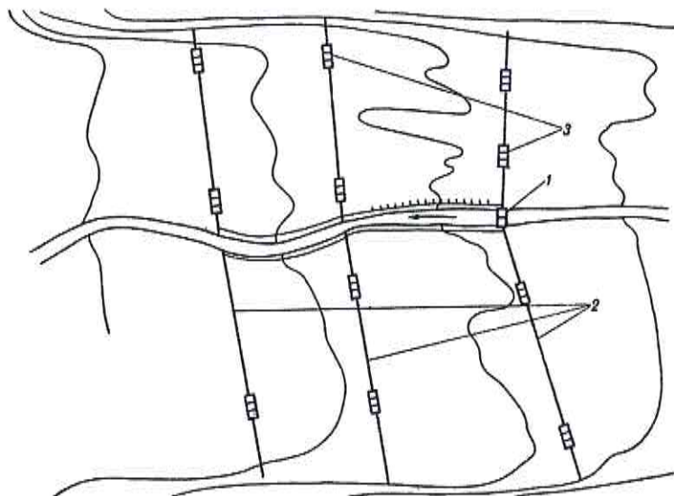
1 – разборная водоподъемная плотина; 2 – валы лиманного орошения; 3 – пропускные шлюзы-регуляторы
