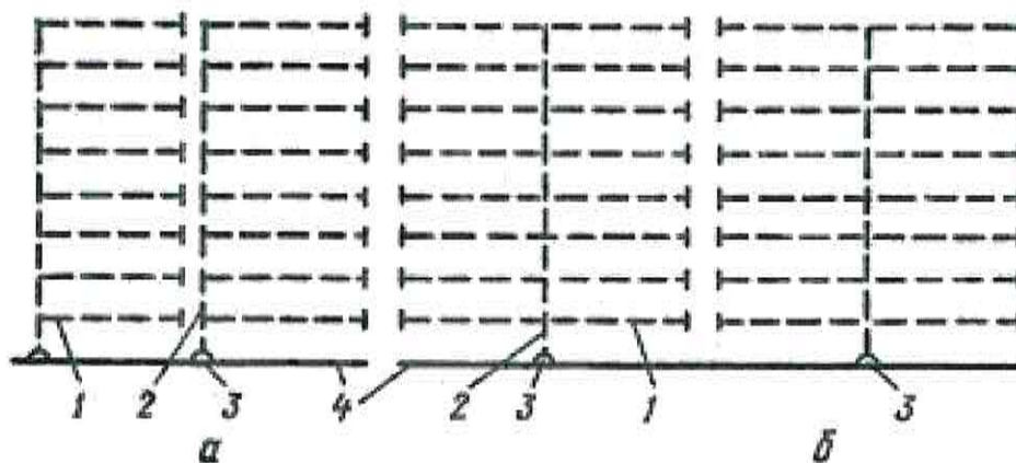
Рисунок Ш.1 – Схемы расположения закрытой регулирующей сети в плане
