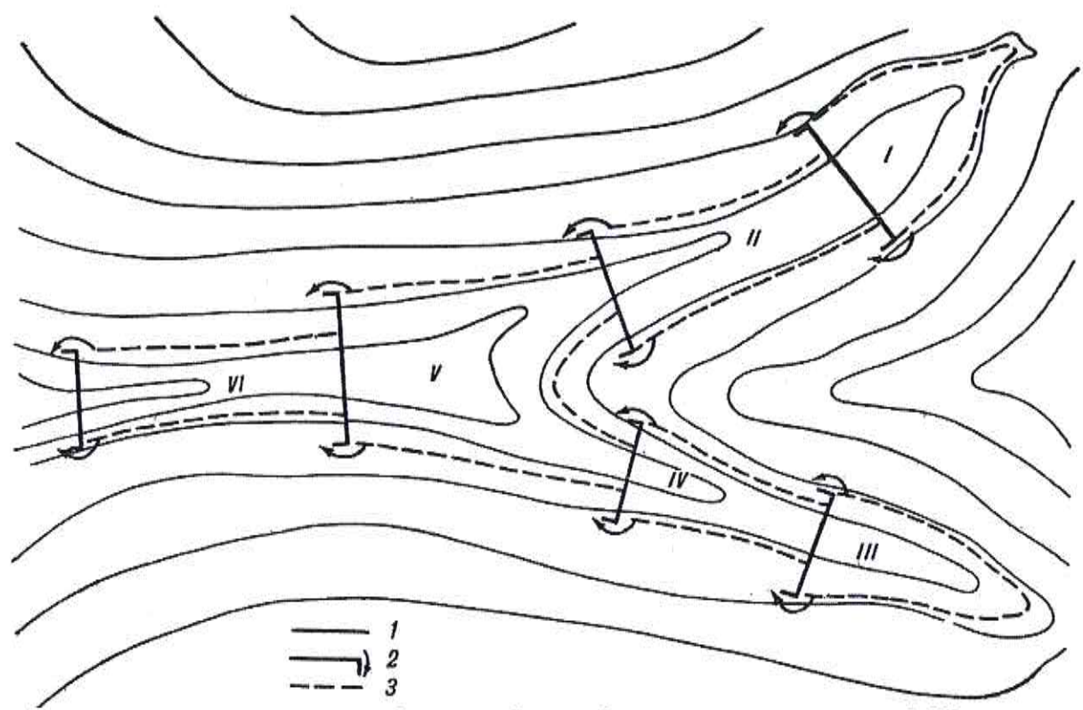
1 – водоудерживающие валы; 2 – водообходы; 3 – границы затопления; I–VI – ярусы
