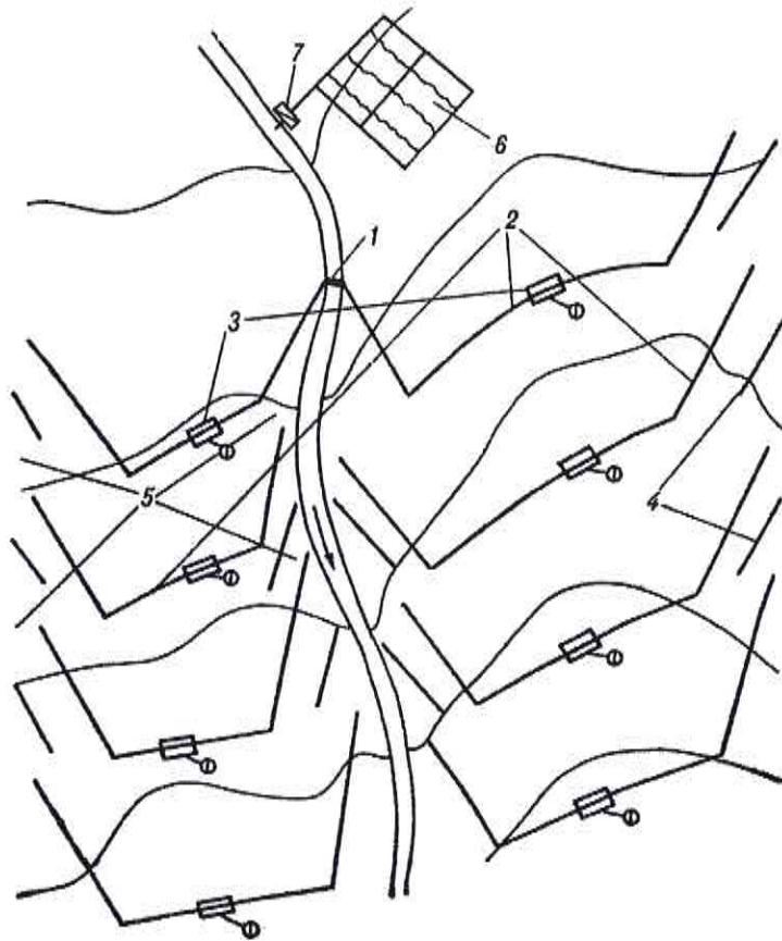
1 – земляная водоподъемная плотина; 2 – земляные валы лиманного орошения; 3 – водовыпуски для опорожнения лиманов; 4 – струенаправляющие валики; 5 – водообходы; 6 – участок регулярного орошения; 7 – насосная станция Рисунок Л.9 – Система ярусных лиманов глубокого слоя затопления, использующая сток степной реки
