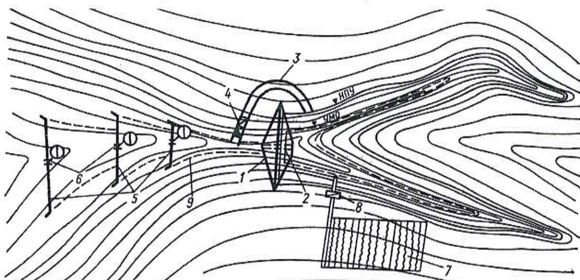
Рисунок Л.7 – Система ярусных лиманов мелкого слоя затопления, питаемая сбросными водами из водохранилища
