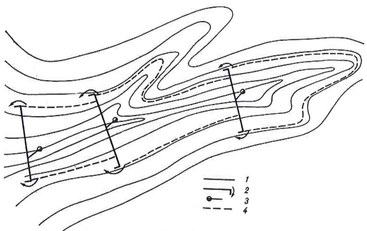
1 – водоудерживающие валы; 2 – водообходы; 3 – сооружения, предназначенные для опорожнения ярусов глубокого затопления; 4 – границы затопления
